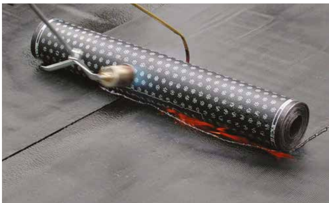
6 pav. Ištirpintos polimerinės – bituminės masės „banga“
