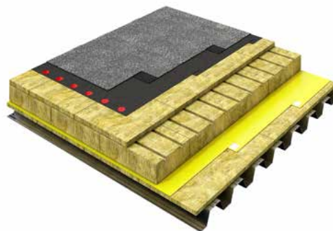
10 pav. Konstrukcija iš dviejų sluoksnių mineralinės šilumos izoliacijos
