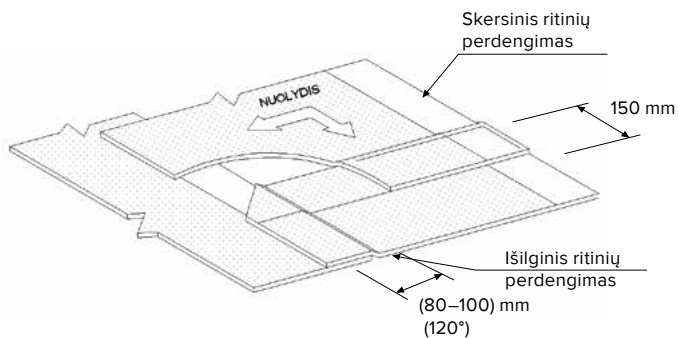
2 pav. Ritinių dangų perdengimas tvirtinant medžiagas mechanškai
